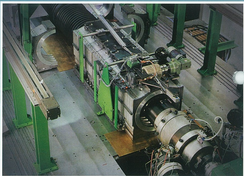
△ ソケット部インライン成形機 HP700型（上部）
